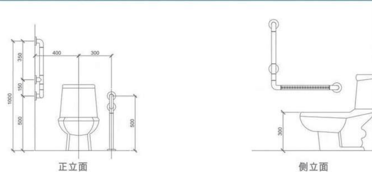
儿童无障碍安装图
